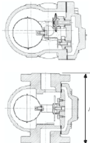
GTF Versione Flangiato / Flanged Version
